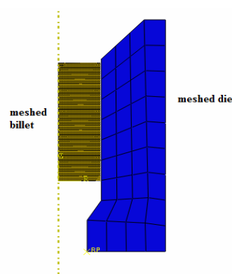
Fig. 3. FEM model
